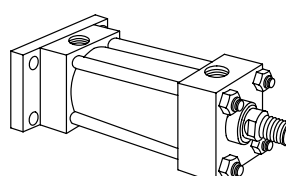
Code 12 Cap rectangular flange ANSI MF2 & ME4
