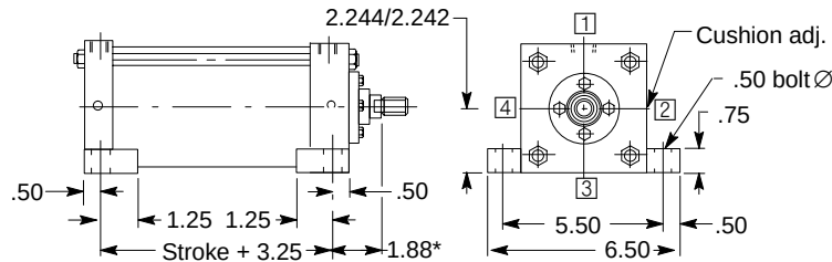
CODE 01 SIDE LUG MOUNT
