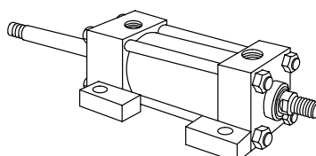
Code 25 Double rod, side lug
